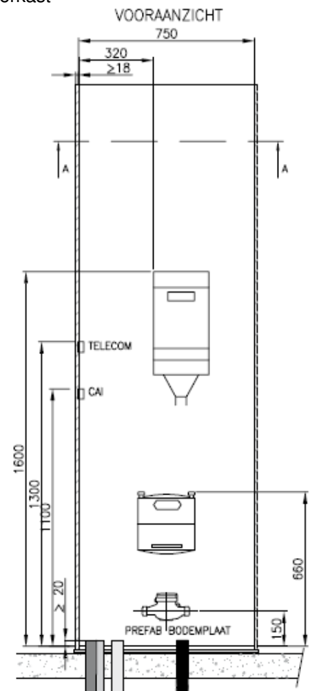
Figuur 2 Vaste afmetingen.
