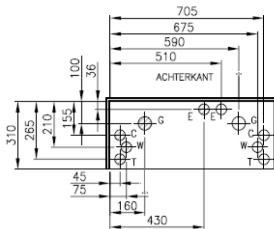
Figuur 1 Kant-en-klare bodemplaat.
