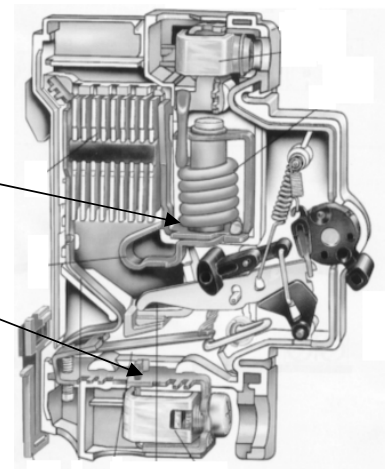
Figuur 7 Binnenwerk installatieautomaat.
