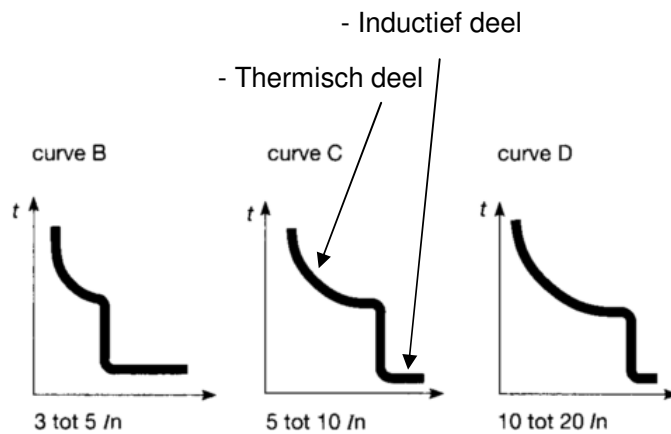
Figuur 8 Uitschakel karakteristiek.
